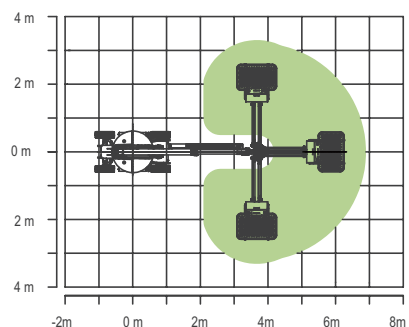
Rozsah rotace platformy ZA10RJE
