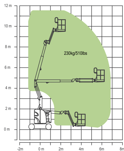
Rozsah pohybu ZA10RJE
